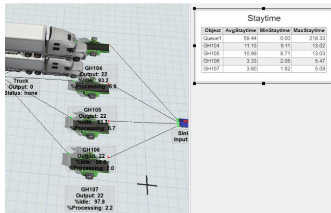
ภาพที่ 14 ผลการจำลองสถานการณ์แนวทางที่ 2
