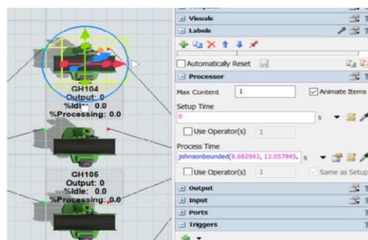
ภาพที่ 6 การกำหนดค่าของ Object Processor (ก่อนปรับปรุง)
