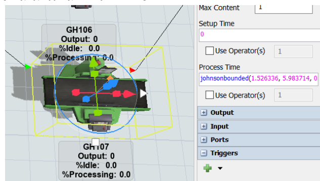
ภาพที่ 16 การกำหนดค่าของ Object Processer ตู้ GH105, GH106, GH107 แนวทางที่ 3
