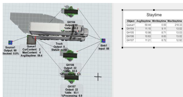
ภาพที่ 8 จำนวนคิวที่เกิดขึ้นและเวลาการให้บริการของตู้ให้บริการ
