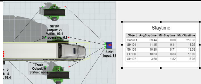
ภาพที่ 11 ผลการจำลองสถานการณ์แนวทางที่ 1
