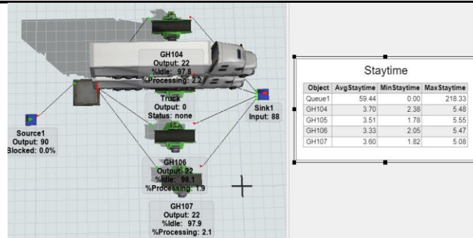
ภาพที่ 20 ผลการจำลองสถานการณ์แนวทางที่ 4
