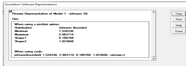
ภาพที่ 4 การแจกแจงระยะเวลาการให้บริการของตู้ออกบัตร (หลังการปรับปรุง)
